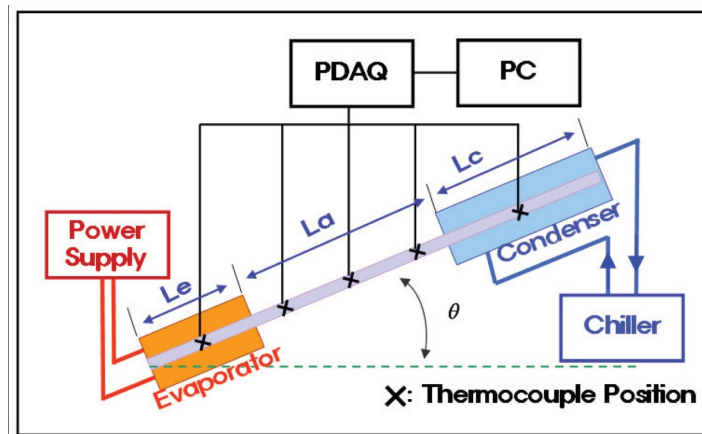
Qmax Test Apparatus
